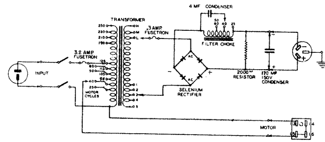
SCHEMATIC WIRING
