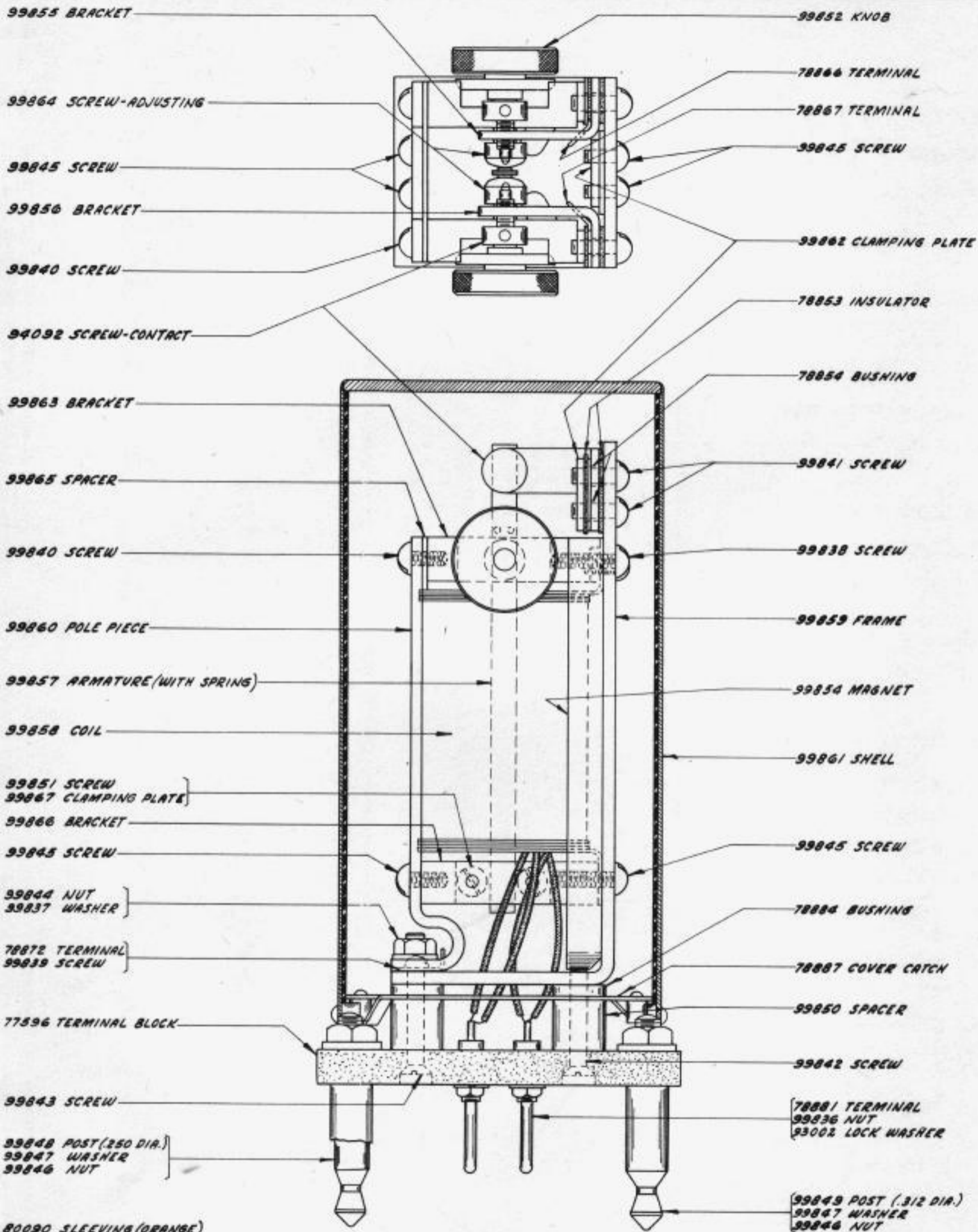
RY-30 LINE RELAY (W.E.CO. 255-A)
